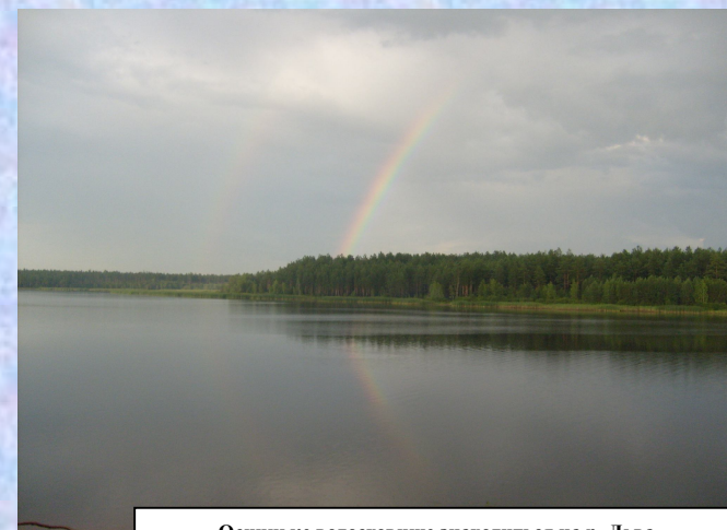
Осиницьке водосховище знаходиться на р. Льва між с. Осинок та с. Старики на трасі Київ-Ковель. Площа дзеркала водосховища при НПУ – 166га; Об'єм води: при НПУ – 3,5млн.м.куб., при УМО – 0,15млн.м.куб. Глибина при НПУ: сер. – 2,0м., макс. – 6,0м.
